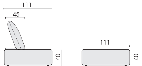
Seitenansicht, Sitzelement, tief (mit Rücken Typ 611)
